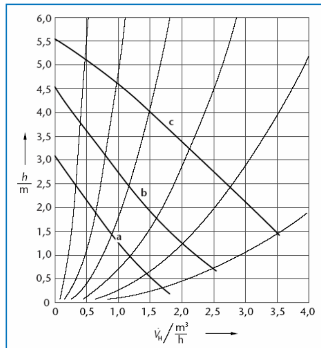
64/2 Характеристики сетевых насосов Star-RS 25/6 и Star-RS 30/6; легенда к рисунку → 64/3
