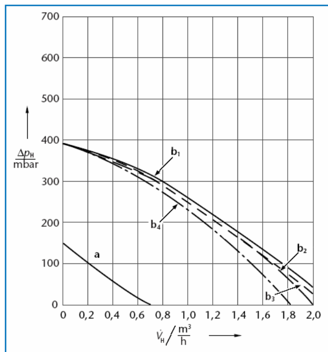
69/1 Остаточный напор систем быстрого монтажа RK 1/G134 и RK 1-E/G134 (→ 21/1)
