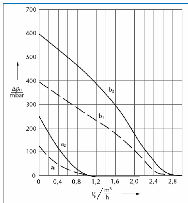
72/3 Остаточный напор систем быстрого монтажа RK 2M(25)/W и RK 2M-E(25)/W для настенной установки (→ 47/1)
