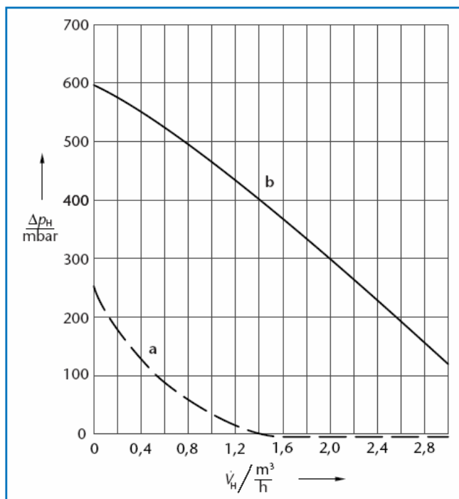
72/2 Остаточный напор системы быстрого монтажа RK 1M-E(32)/W для настенной установки (→ 47/1)
