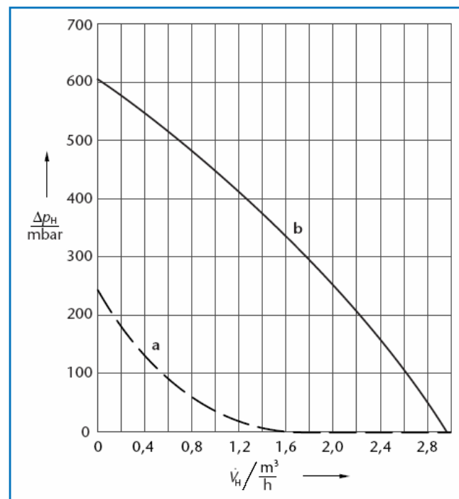
70/4 Остаточный напор системы быстрого монтажа RK 2M-E(32)/G215 (→ 37/1)
