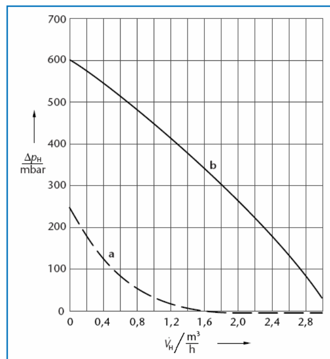
70/2 Остаточный напор системы быстрого монтажа RK 1M-E/G215 (→ 37/1)
