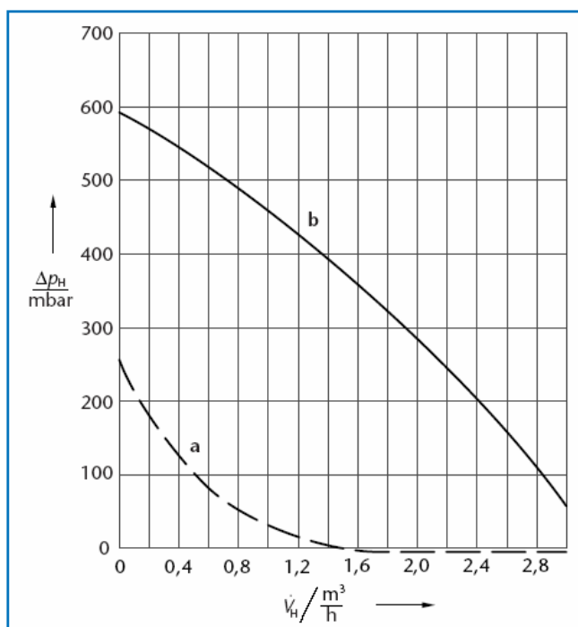
72/4 Остаточный напор системы быстрого монтажа RK 2M-E(32)/W для настенной установки (→ 47/1)
