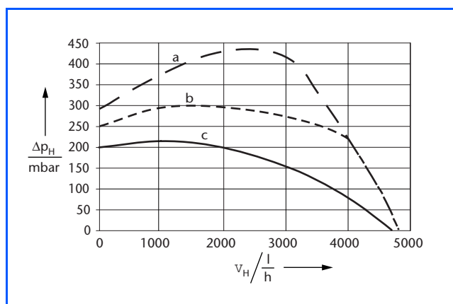
33/3 Остаточный напор отдельного насоса WILO TOP-E 25/1-7
