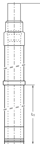
Коаксиальный патрубок из нержавеющей стали для подачи приточного воздуха
