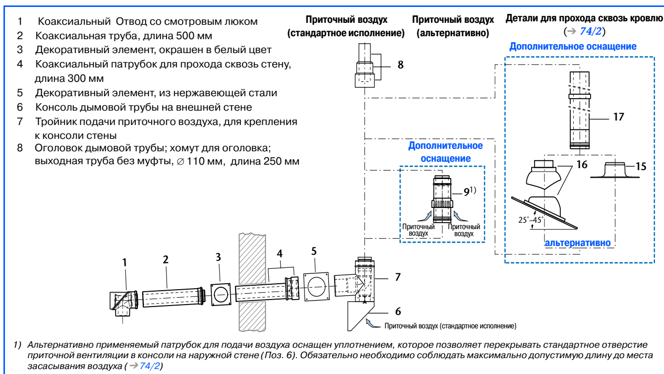
75/1 Детали основного монтажного комплекта GAF-K из пластика для котлов Logamax plus GB 162
