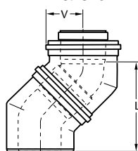
Размеры смещения коаксиального колена
