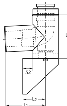
Концентрический тройник из нержавеющей стали (в основном монтажном комплекте GAF-K)
