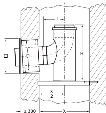
Соединение коллектора с дымовой трубой
