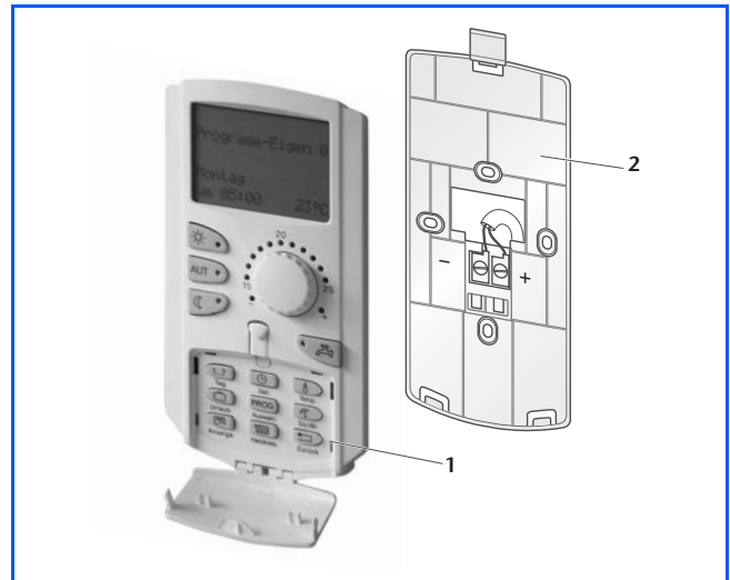
26/1 Блок управления MEC2 с интегрированным датчиком температуры в помещении и настенным креплением
