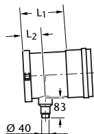
Закрывающая деталь коллектора с конденсатоотводчиком
