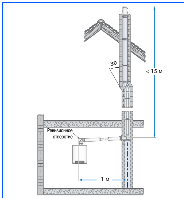
67/1 Пример расположения отверстия для чистки горизонтального дымоотвода трубопроводе без поворотов в котельном помещении
