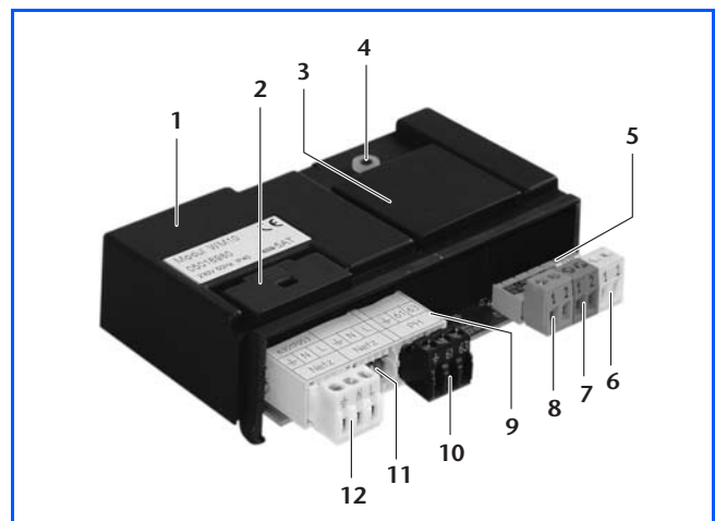
20/1 Модуль гидравлической стрелки WM10
