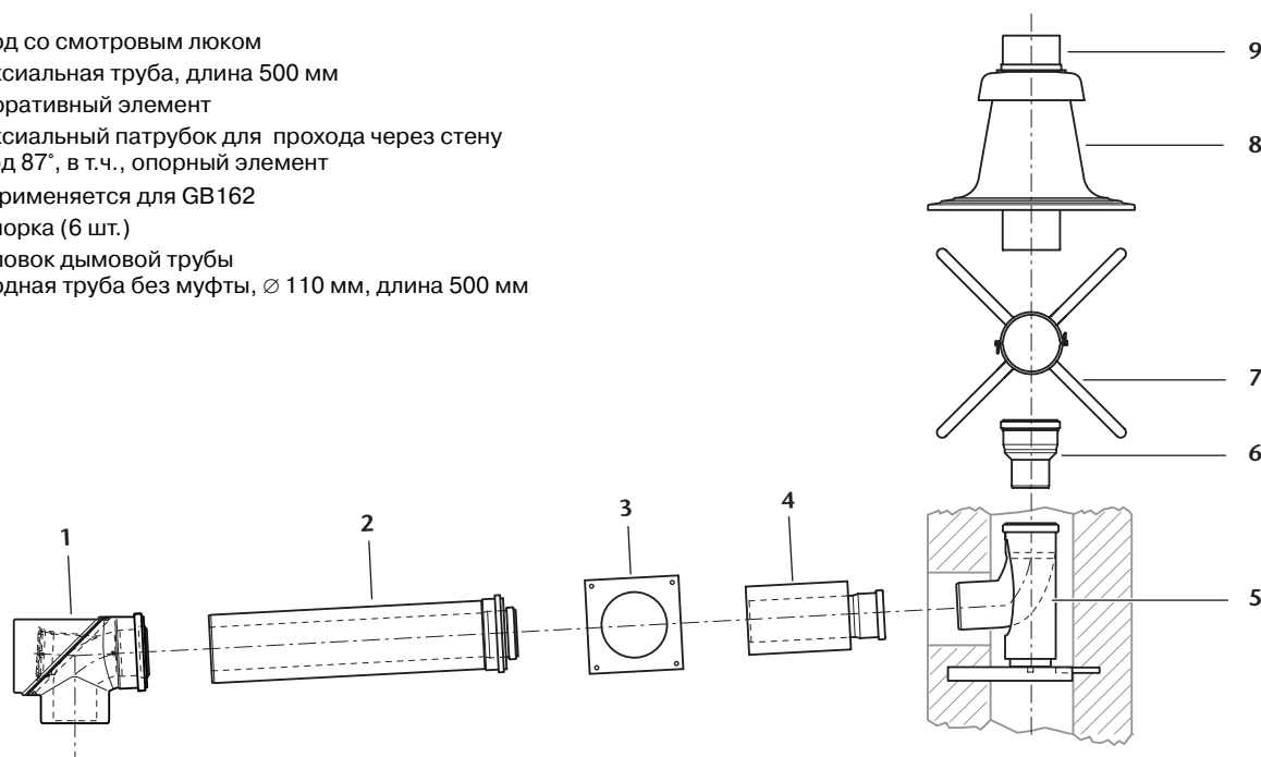
71/1 Детали основного монтажного комплекта GA-K из пластика для колов Logamax plus GB162
