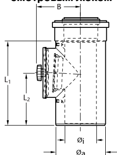
Концентрическая труба со смотровым люком
