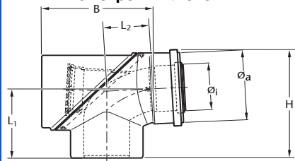
Концентрический отвод со смотровым люком
