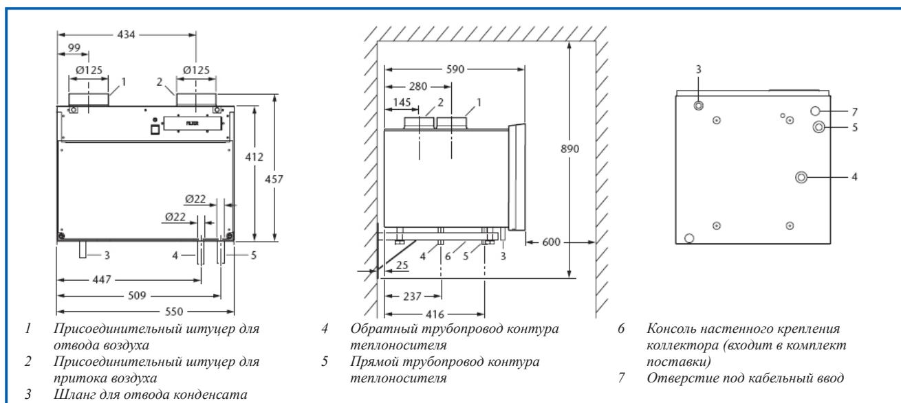
69/1 Монтажные размеры коллектора отработавшего воздуха помещений (AK) (размеры указаны в мм)
