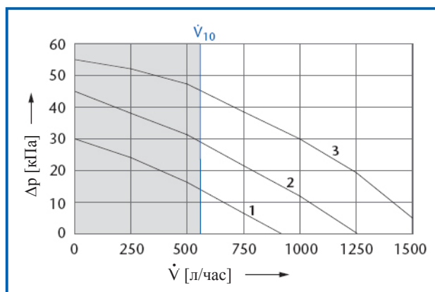
57/4 Отопительный насос WPS 6 K
