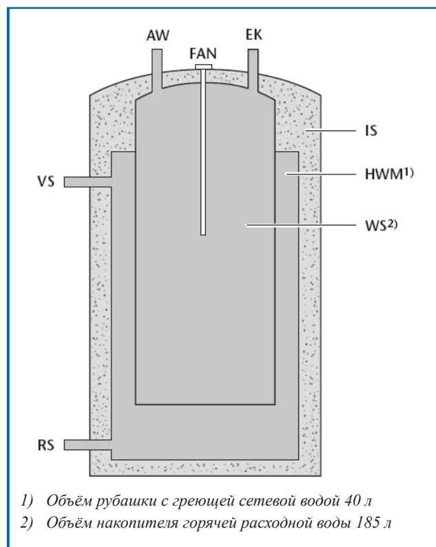
42/2 Устройство бойлера-накопителя из высококоротной стали
