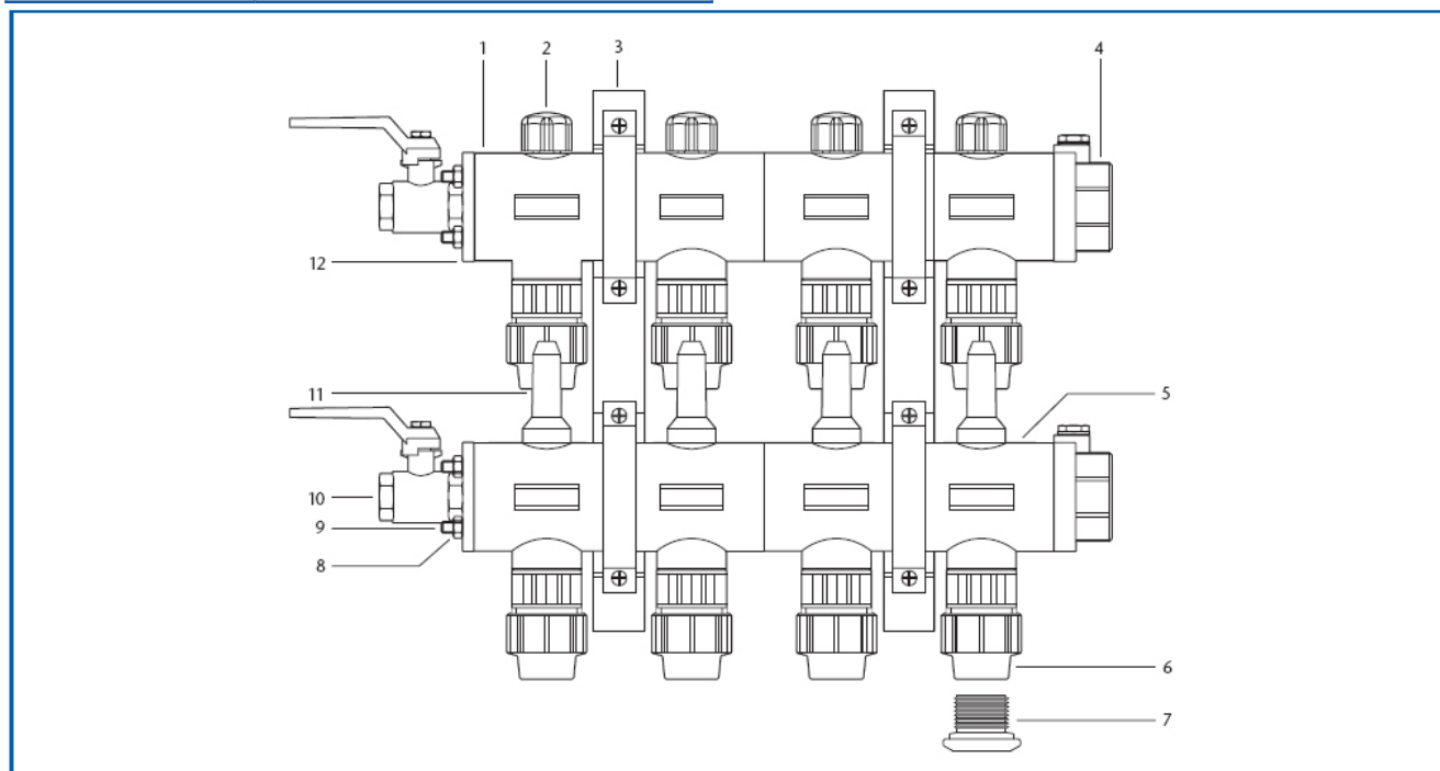
75/2 Устройство распределителя рассольного контура. Пример для 4-х рассольных контуров.
