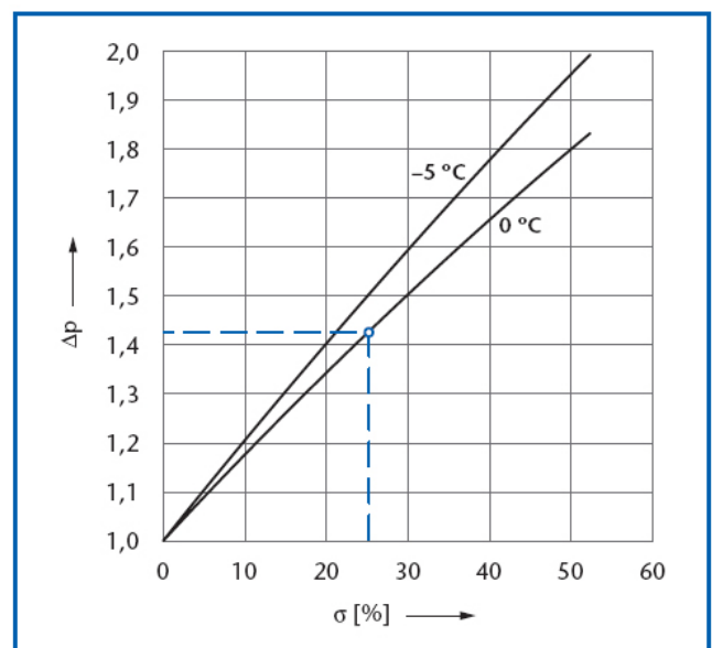
35/2 Относительная потеря давления водно-моноэтиленгликолевых смесей в сопоставлении с водой в зависимости от концентрации
