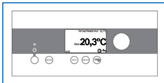
36/1 Регулятор HMC10
