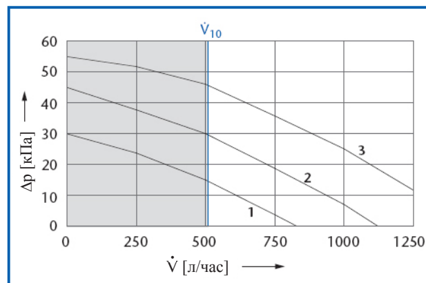
57/2 Отопительный насос WPS 6
