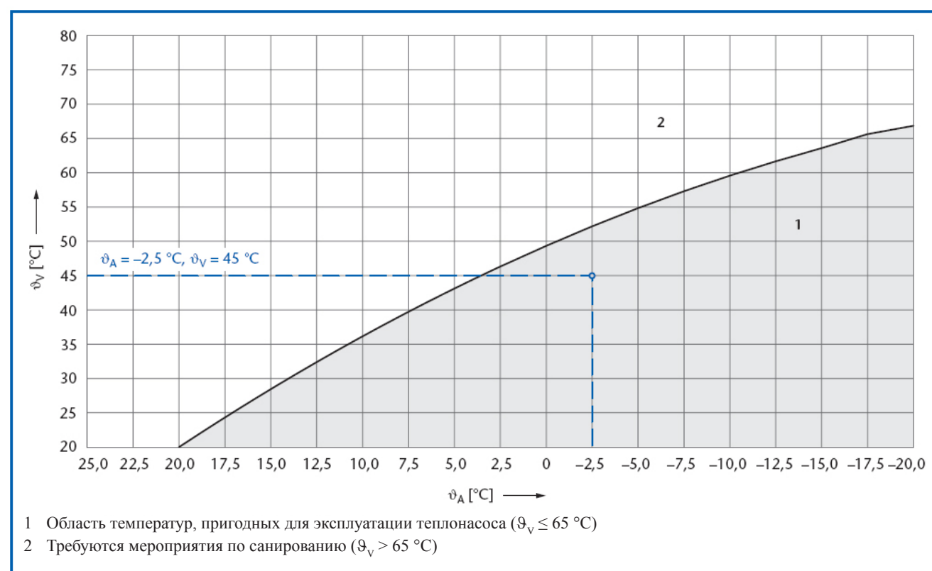
III/2 Диаграмма для определения требуемых системных температур
