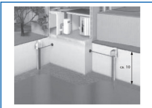
8/2 Колодцы грунтовых вод (размеры указаны в метрах)
