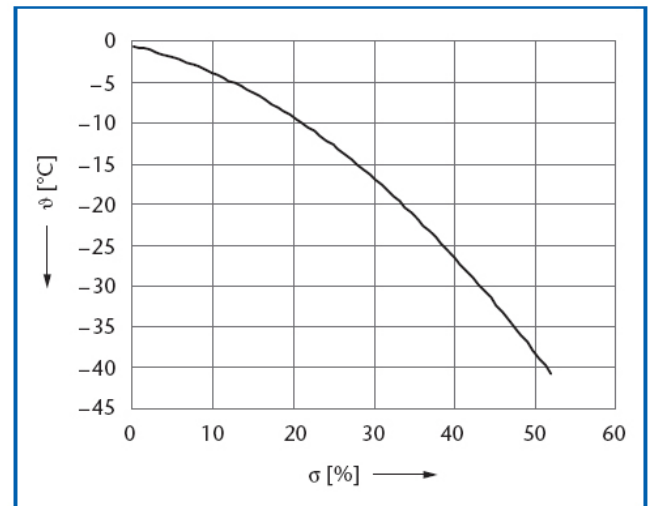
19/1 Температурная кривая замедления смеси моноэтиленгликоль / вода в зависимости от концентрации
