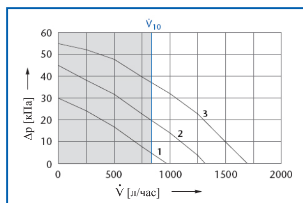
57/6 Отопительный насос WPS 9
