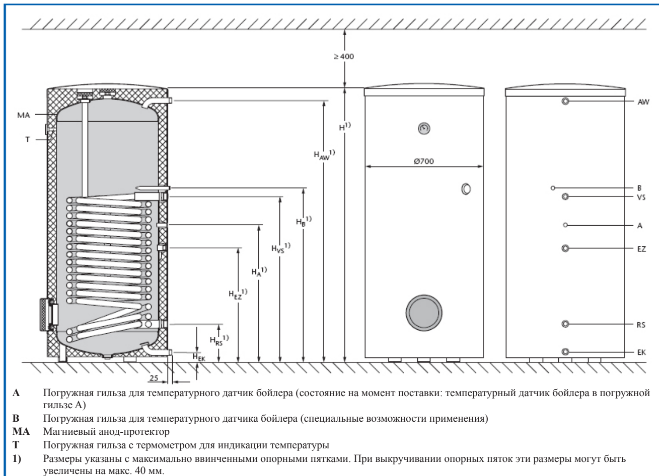
61/1 Монтажные размеры бойлеров SH 290 RW, SH 370 RW и SH 450 RW (размеры указаны в мм)
