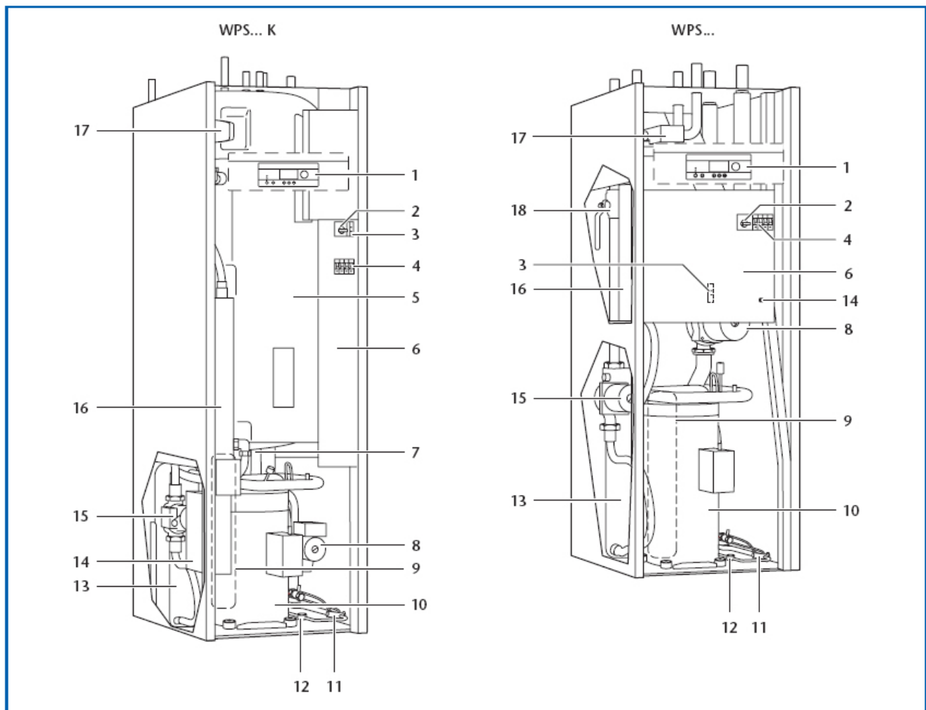
35/1 Устройство теплового насоса
