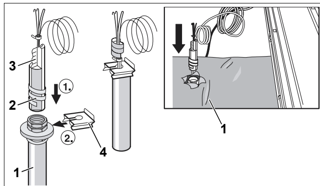
Рис. 30 Установка комплекта температурных датчиков
