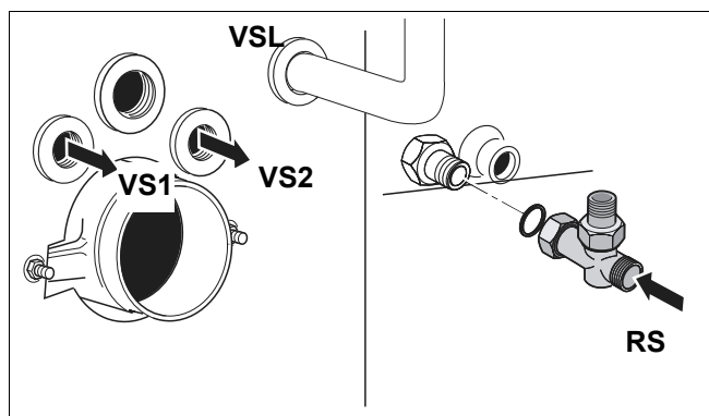
Рис. 21 Подключение бака-водонагревателя
