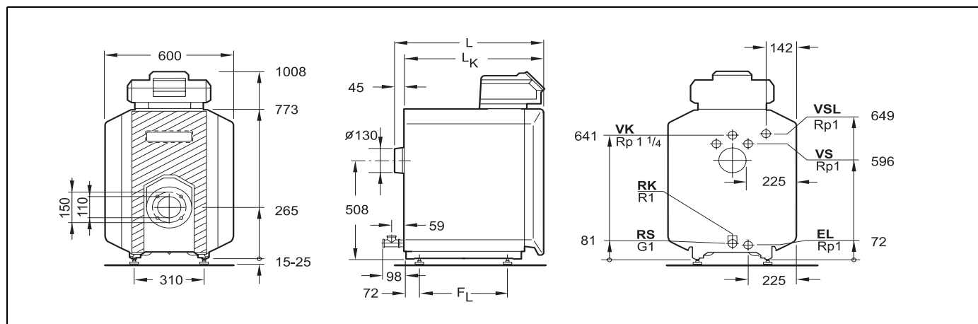
Рис. 2 Подключения и размеры (приведены в мм)
