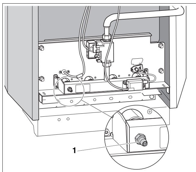
Рис. 44 Газовая горелка
