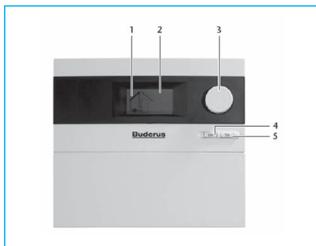
29/1 Гелиотерморегулятор Logamatic SC20
