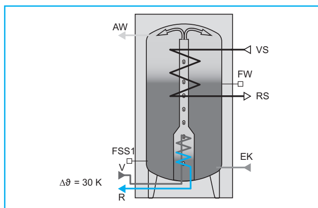
23/2 Нагрев термосифонного бойлера до \Delta\theta = 30\text{ K} во время интенсивной инсоляции путем регулирования оборотов насоса в режиме повышенного расхода (High-Flow)
