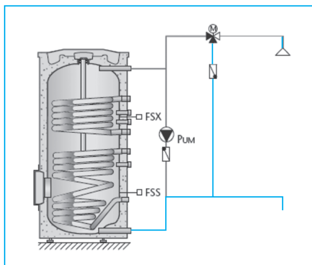
27/1 Температурное перераспределение (рециркуляция) в схеме с одним гелиобойлером
