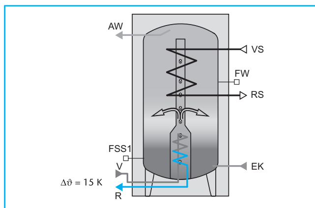
23/1 Приоритетный нагрев зоны готовности термосифонного бойлера до \Delta\theta = 15\text{ K} частным регулированием оборотов насоса в режиме уменьшенного расхода (Low-Flow), достижение температуры 45 °C в районе граничного термодатчика FW
