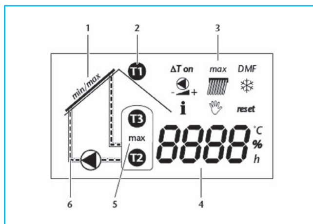
29/2 Сегментированный жидкокристаллический дисплей гелиотерморегулятора Logamatic SC20
