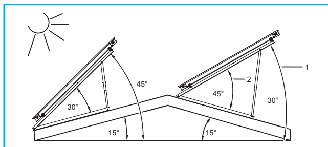
111/1 Примеры фактических углов наклона при использовании рам для установки гелиоколлекторов на плоской крыше с незначительным уклоном ( <25^\circ )
