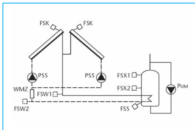
37/1 Регулирование «восток/запад» через две комплексные гелиостанции
