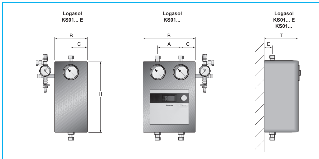
41/1 Габаритные размеры комплексных гелиостанций Logasol KS...
