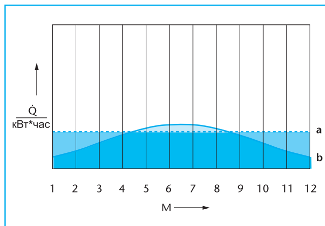
4/1 Соотношение между выработкой энергии гелиоколлекторной установкой и годовой потребностью в тепловой энергии для ГВС
