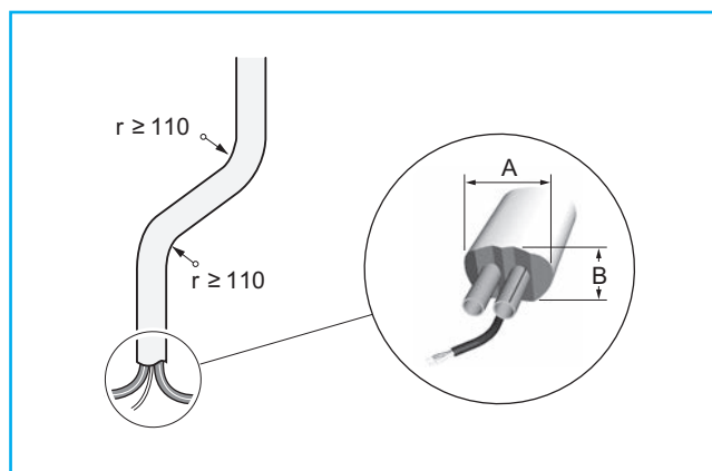
42/2 Минимальный радиусгиба для Twin-Tube 15 (габаритные размеры → 43/1)
