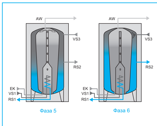
18/3 Пополнение накопителя холодной воды с помощью теплообменника гелиоконтура и буферного аккумулятора горячей воды (5), а также дополнительный нагрев от обычного котла отопления в случае недостаточного количества гелиотермической энергии (6)
