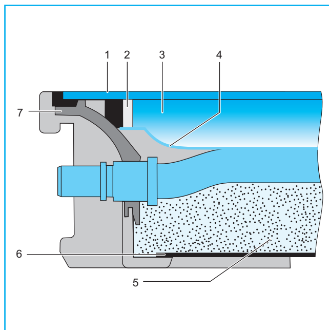
10/1 Вид в разрезе высокопроизводительного плоского гелиоколлектора Logasol SKS4.0 с заполнением инертным газом
