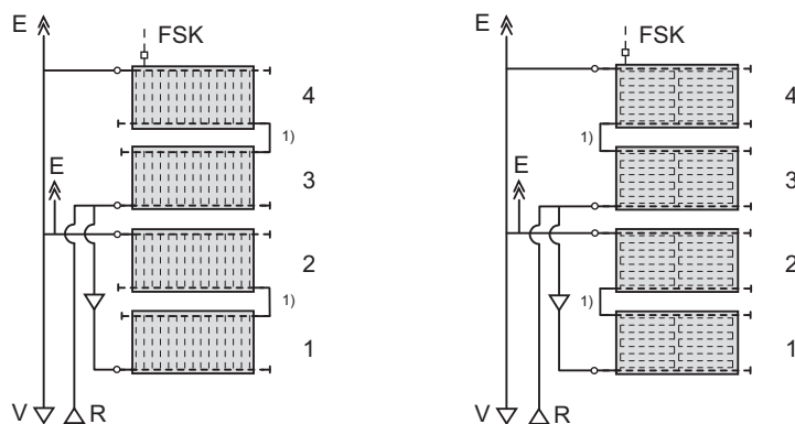
86/1 Схема подключения более трех гелиоколлекторов горизонтального типа, расположенных один над другим
