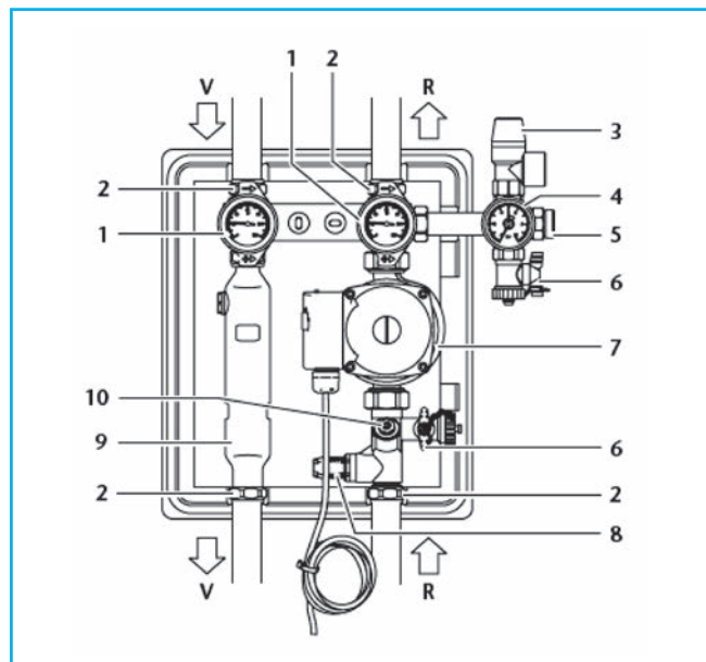
40/1 Устройство комплексной гелиостанции Logasol KS01.. без интегрированного гелиотерморегулятора
