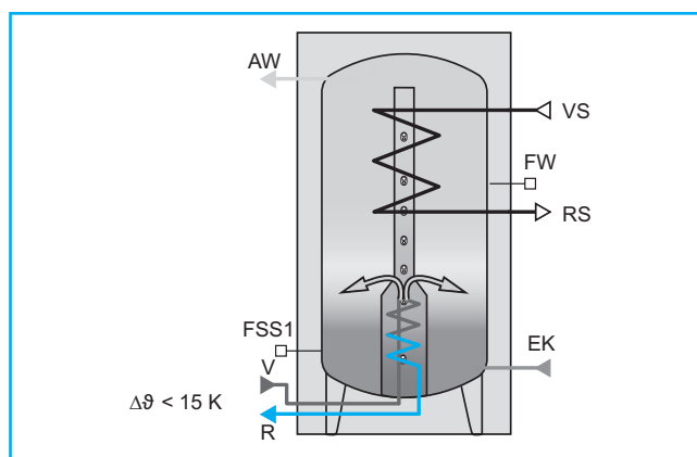
23/3 Нагрев термосифонного бойлера с максимально возможной температурой в подающем трубопроводе ( \Delta\theta < 15\text{ K} ) путем регулирования оборотов насоса во время малой инсоляции
