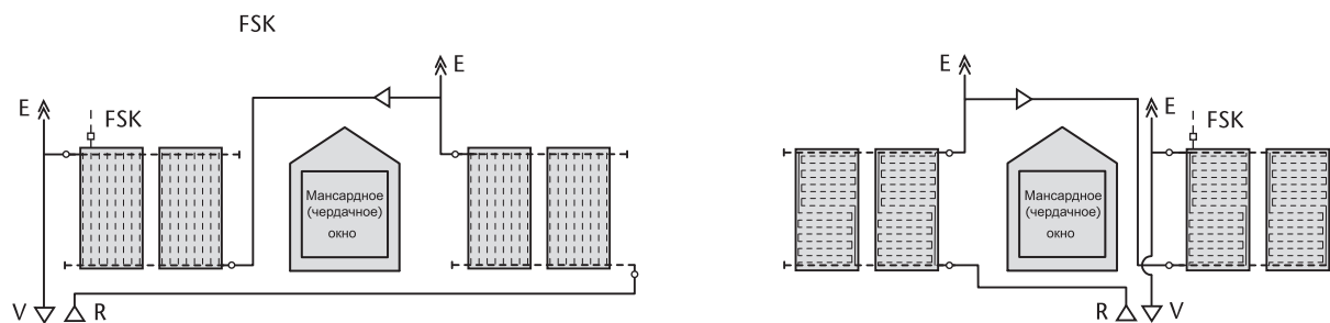
86/2 Гидравлика гелиоколлекторов для монтажа на крыше с мансардным (чердачным) окном
