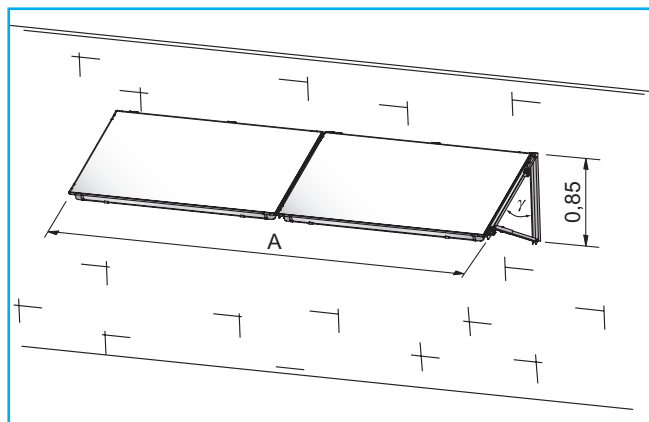
82/1 Монтажные размеры фасадных комплектов для плоских гелиоколлекторов Logasol SKN4.0-w и SKS4.0-w горизонтального типа; (размер A в м, → 82/2)
