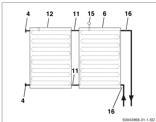
Рис. 62 Гидравлические подключения
