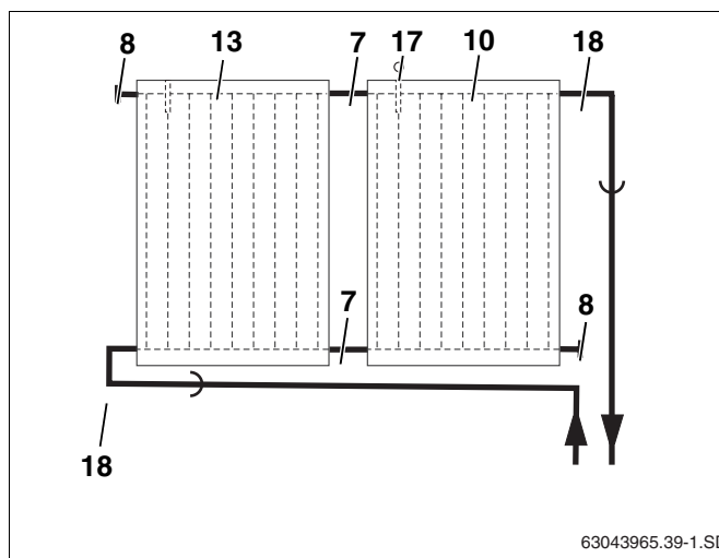
Рис. 62 Гидравлические подключения
