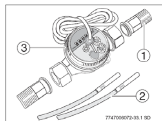
Рис. 6 Тепловой счётчик
