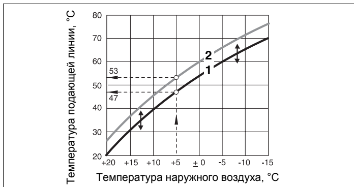
Рис. 2 Отопительная кривая (пример), до повышения заданной температуры помещения на 2^{\circ}\text{C} (1) и после него (2)
