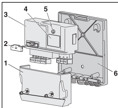
Fig. 1 Overzicht EM10 pos. 1: Beschermkap pos. 2: Zekeringhouder pos. 3: Module EM10 pos. 4: Typeplaatje pos. 5: Bedrijfs-/storing LED pos. 6: Wandhouder
