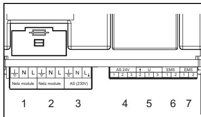
Obr. 2 Prípojky poz. 1: 230V-sieťová prípojka poz. 2: 230V-prípojka pre 2. Modul poz. 3: Výstup alarmu 230V poz. 4: Výstup alarmu 24V poz. 5: Riadiaci signál 0-10V poz. 6: Vstup zbernice EMS poz. 7: Výstup zbernice EMS
