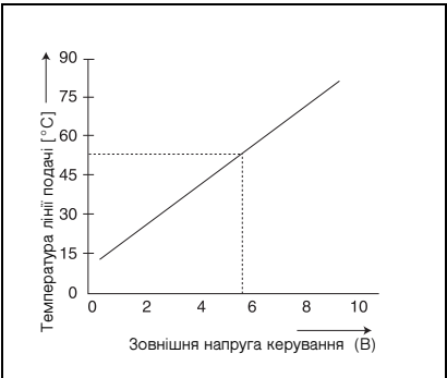
мал. 3 0 – 10В діаграма
