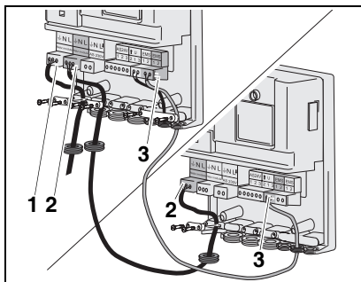
мал. 4 З'єднати між собою два модуля, встановити підключення до мережі
