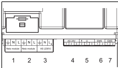
2. ábra Csatlakozások
