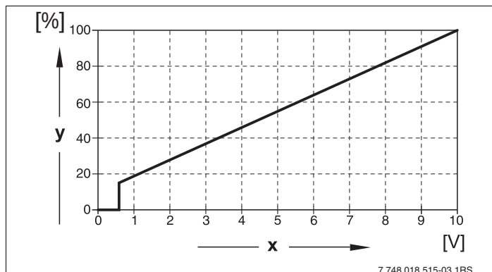
Рис. 11 Вход 0–10 В
