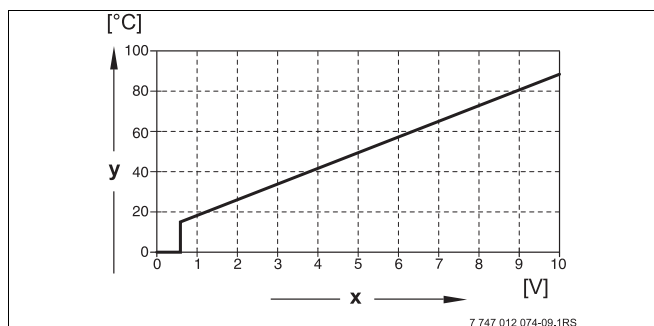
Рис. 10 Вход 0–10 В
