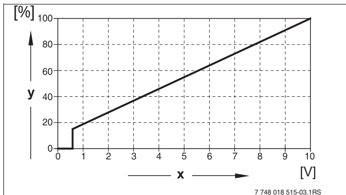
Рис. 2 Вход 0 – 10 В
