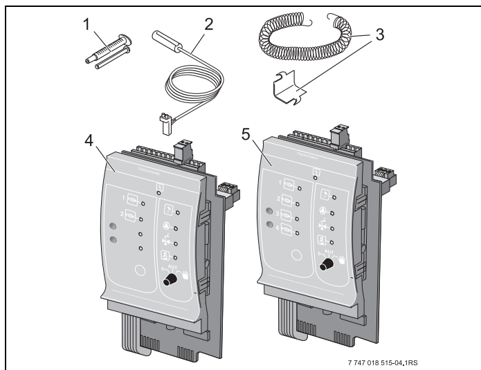
Рис. 4 Комплект поставки функционального модуля FM456/FM457
