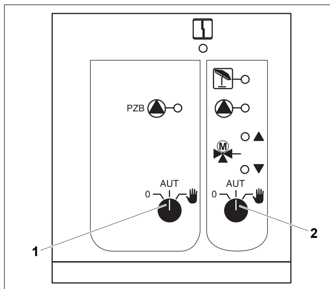
Рис. 26 Центральный модуль ZM433
