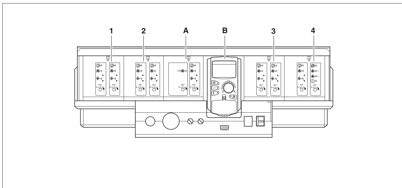
Рис. 5 Оснащение модулями (полная комплектация)
