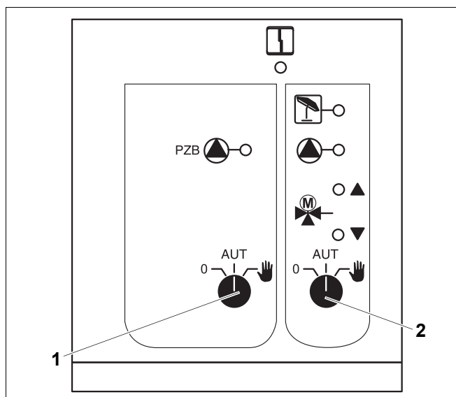
Рис. 22 Центральный модуль ZM433
