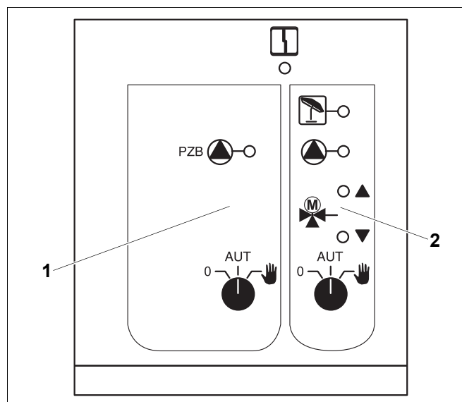
Рис. 21 Центральный модуль ZM433
