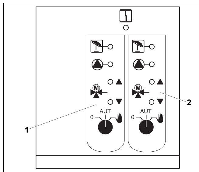
Рис. 25 Функциональный модуль FM442
