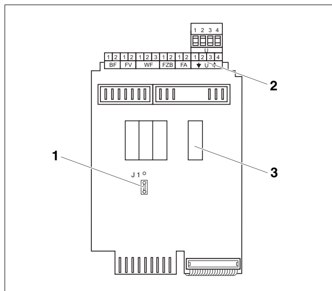
Рис. 9 ZM433 (вид сзади)
