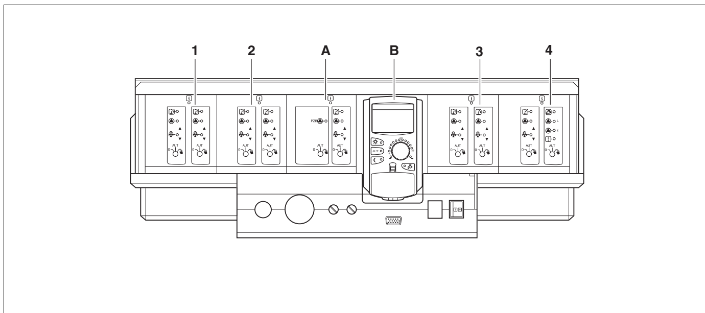
Рис. 3 Комплектация модулями
