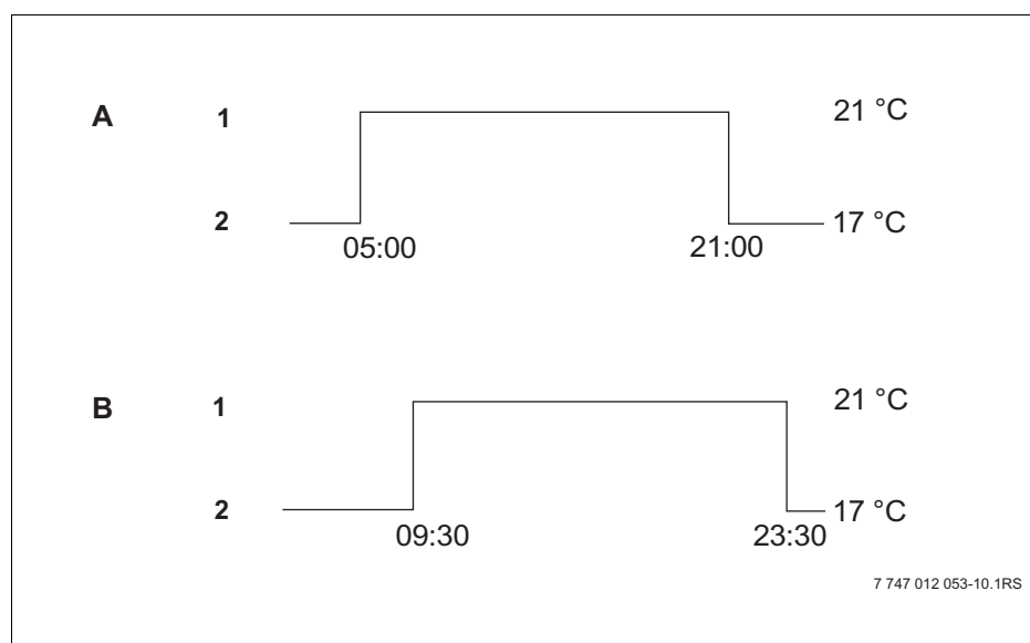
Рис. 19 Новая программа отопления
