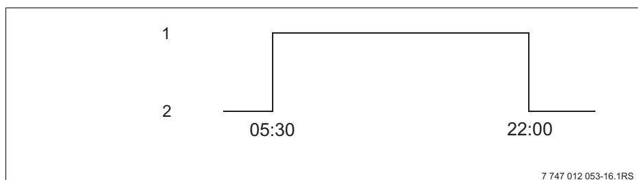
Рис. 11 Пример стандартной программы (здесь: "Программа семья" с понедельника по четверг)
