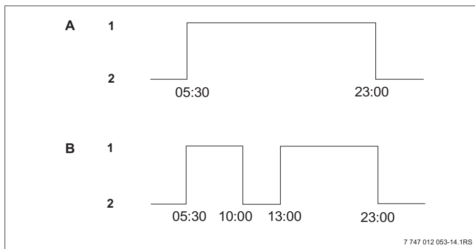
Рис. 15 Ввод времени переключения для прерывания периода отопления
