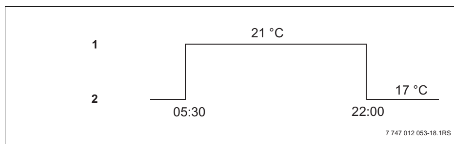
Рис. 8 Смена в заданное время дневного и ночного режимов (пример)
