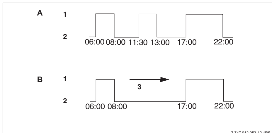
Рис. 17 Отмена отопительного периода
