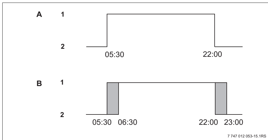
Рис. 13 Изменение времени включения с 05:30 на 06:30 и времени выключения с 22:00 на 23:00 (пример)
