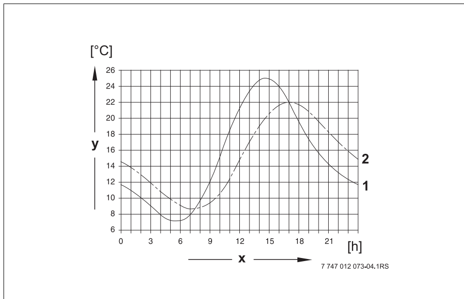
Рис. 14 Сравнение текущей и демпфированной температуры наружного воздуха
