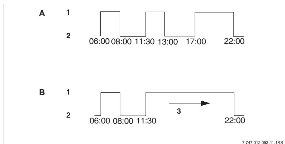
Рис. 18 Объединение двух отопительных периодов
