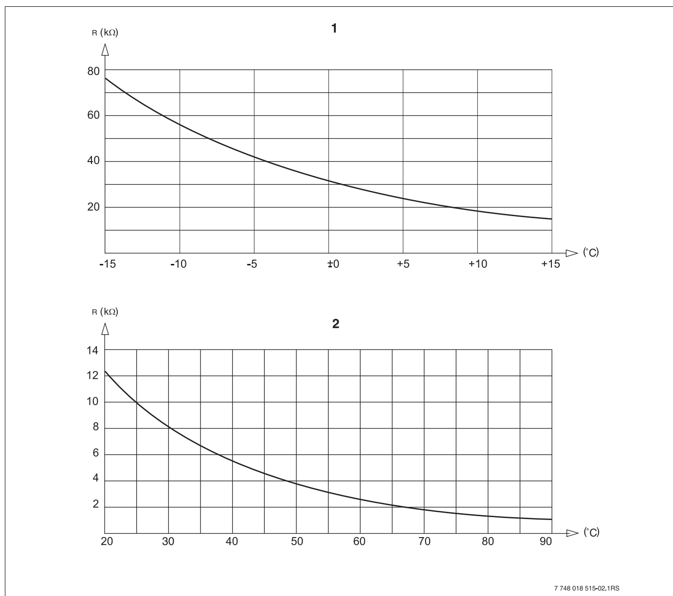
Рис. 17 Датчики наружной температуры, температуры котловой воды, подающей линии, горячей воды
