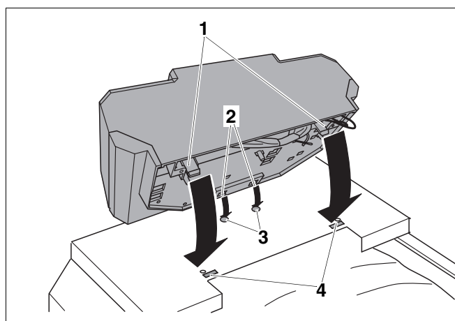
Рис. 62 Установка системы управления
