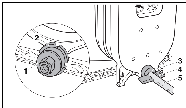
Рис. 18 Установка стяжного инструмента на нижней ступице котла
