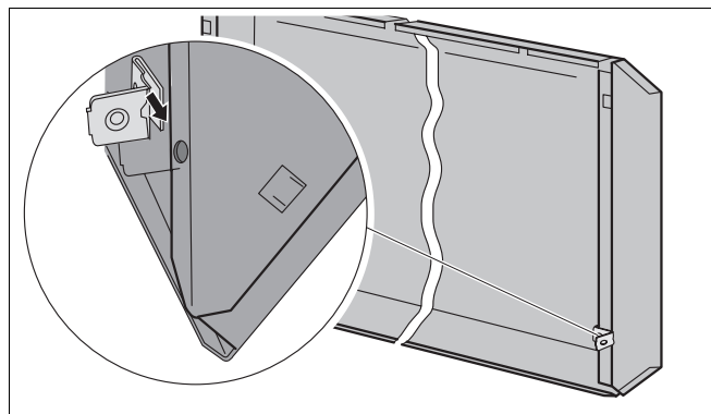
Рис. 44 Установка гайки с защелкой (здесь: на правой стороне)
