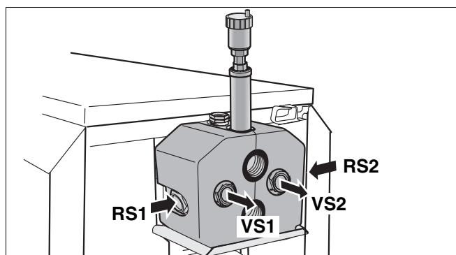
Рис. 58 Подключение бака-водонагревателя
