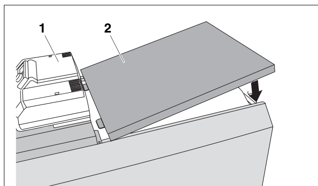
Рис. 67 Установка задней крышки котла
