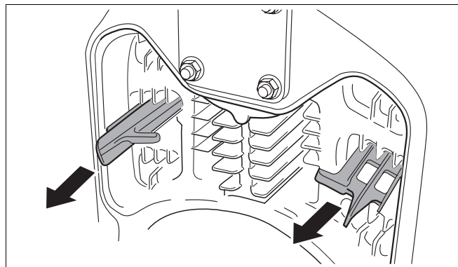
Рис. 70 Удаление направляющих пластин дымовых газов (пример: 2-ой газоотводящий канал)
