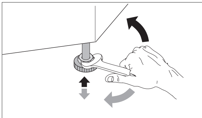
Рис. 53 Выравнивание отопительного котла по горизонтали
