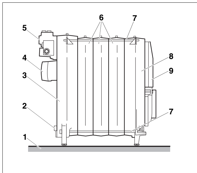
Рис. 8 Смонтированный котловой блок
