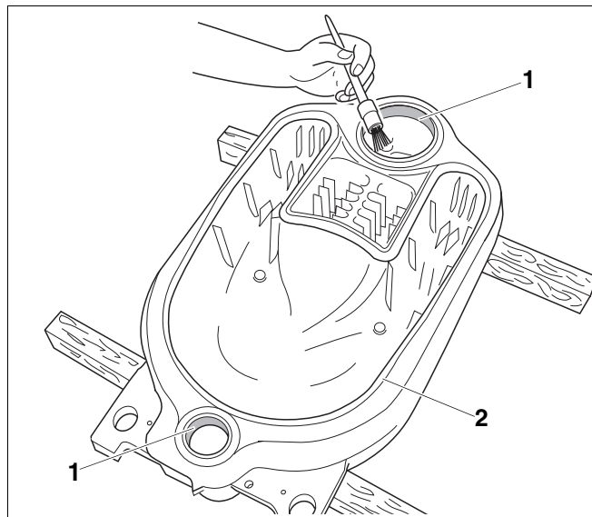
Рис. 10 Нанесение сурика на ступицы котла
