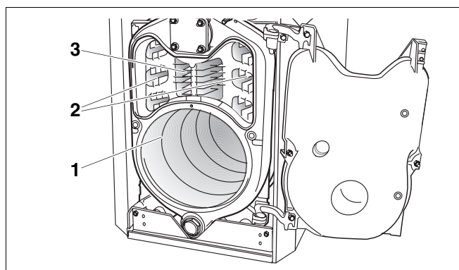
Рис. 77 Открытая дверца горелки
