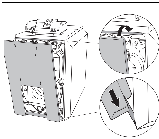
Рис. 73 Установка обшивки дверцы горелки
