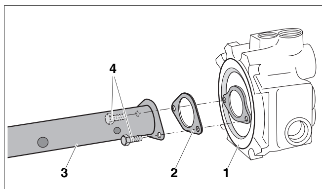
Рис. 22 Установка подпиточной трубы и соединительного элемента
