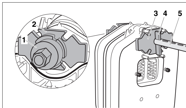
Рис. 17 Установка стяжного инструмента на верхней ступице котла
