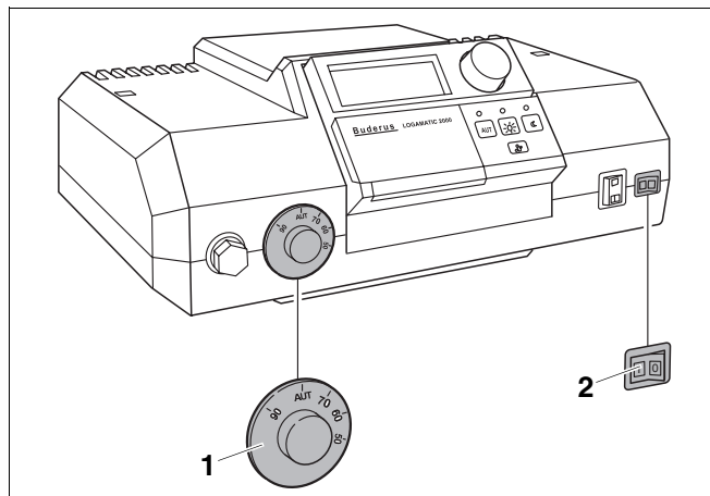
Рис. 69 Включение системы управления (например, Logamatic 2000)
