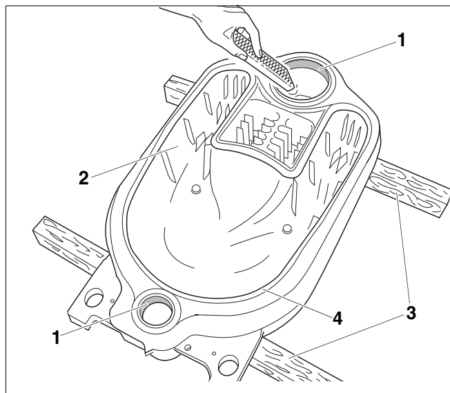
Рис. 9 Удаление заусенцев
