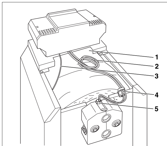
Рис. 64 Прокладка и подключение проводов
