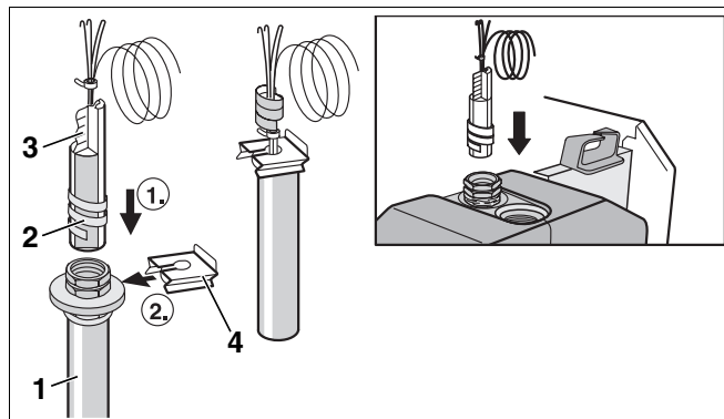
Рис. 65 Установка комплекта температурных датчиков
