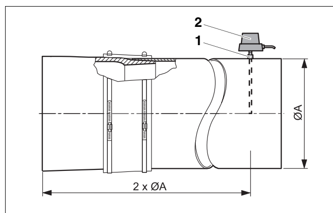
Рис. 55 Установка датчика температуры дымовых газов (принципиальная схема)
