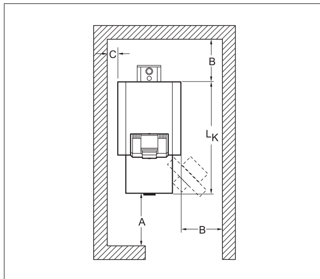
Рис. 7 Расстояния от стен в помещении (котел располагается справа или слева)
