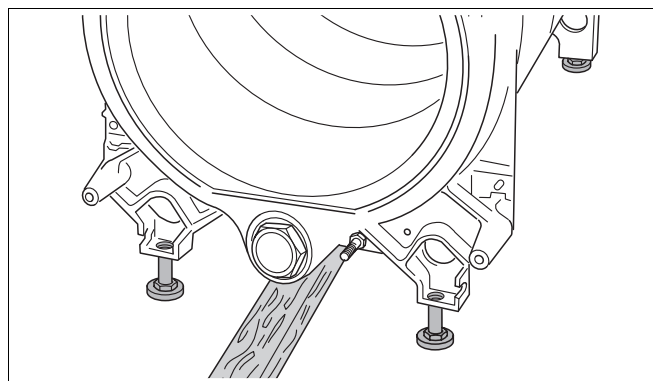
Рис. 33 Установка опорных болтов
