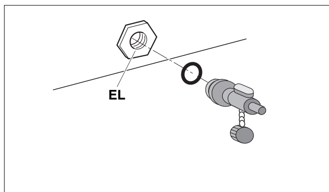
Рис. 59 Установка крана для наполнения и слива
