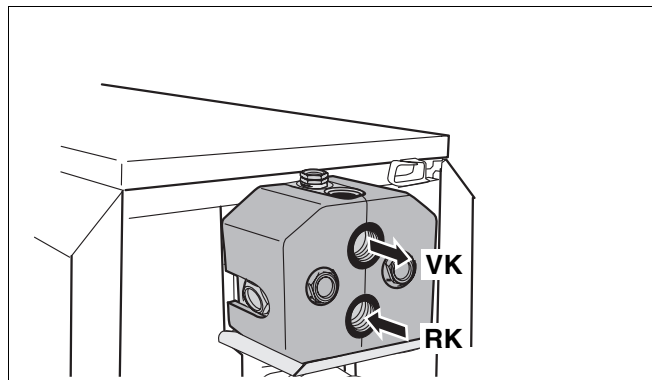
Рис. 56 Подключение подающей и обратной линий отопления
