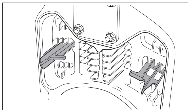
Рис. 34 Укладка направляющих пластин дымовых газов во 2-ой газоотводящий канал (здесь: в середине)
