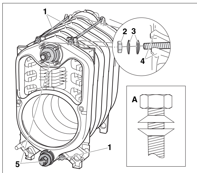
Рис. 21 Установка анкерных штанг – расположение тарельчатых пружин
