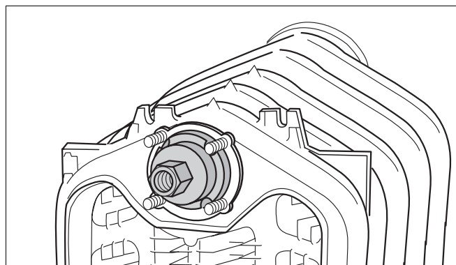
Рис. 20 Установка стяжного инструмента на переднюю секцию котла
