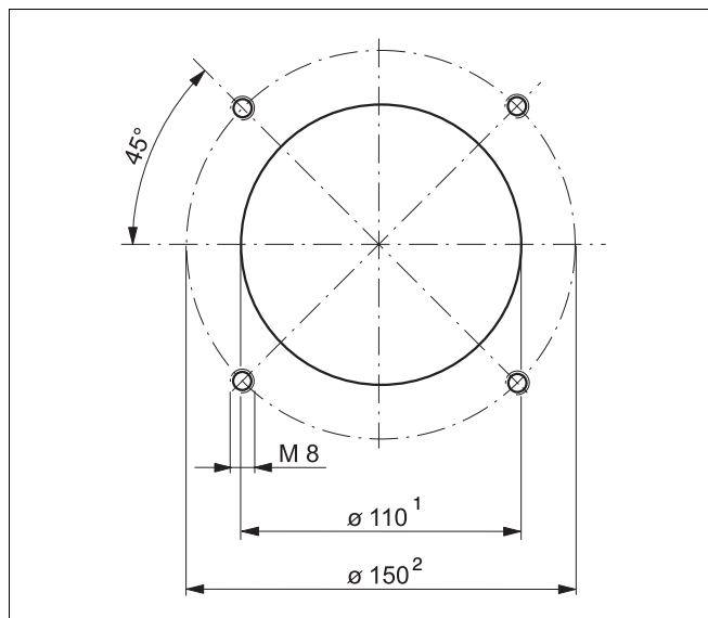
Рис. 61 Окружность с отверстиями на дверце горелки (присоединительный фланец по DIN EN 226, размеры в мм)
