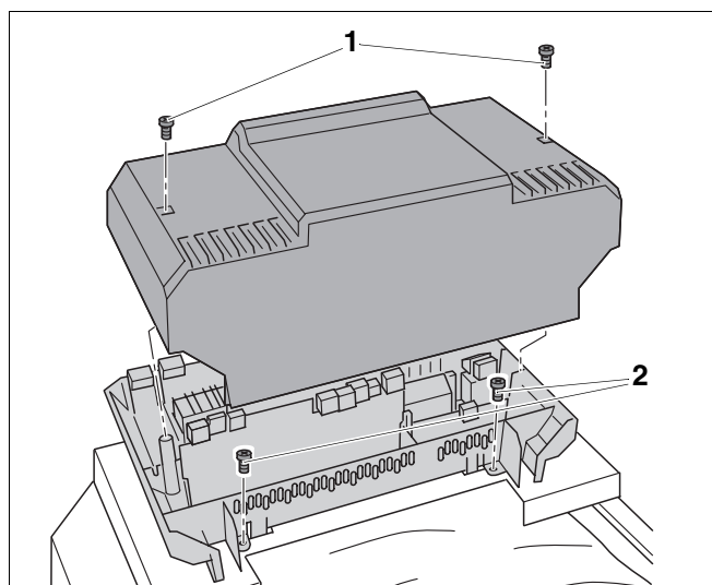
Рис. 63 Снятие верхней крышки
