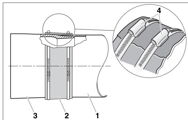
Рис. 54 Установка уплотнительной манжеты дымовой трубы (принципиальная схема)
