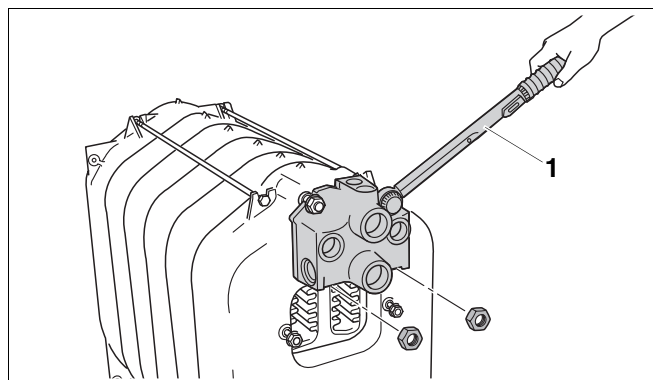
Рис. 24 Установка соединительного элемента
