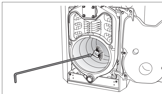
Рис. 79 Чистка топочной камеры
