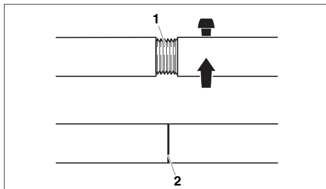
Рис. 16 Резьбовое соединение стяжных штанг
