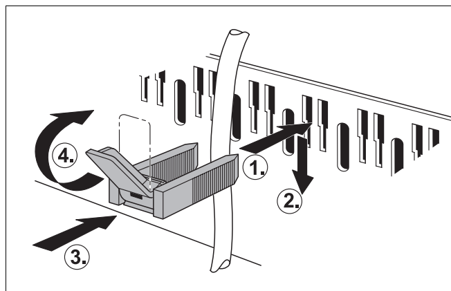
Рис. 66 Крепление проводов хомутами
