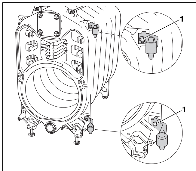
Рис. 36 Монтаж шарнирных крюков (здесь: с правой стороны)
