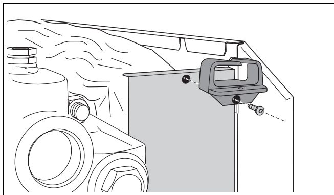
Рис. 49 Монтаж кабельного хомута
