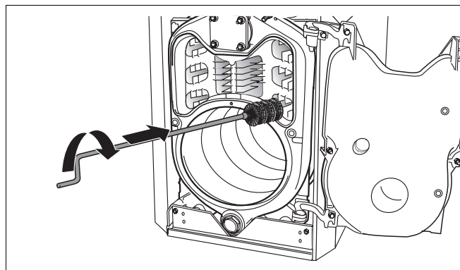
Рис. 78 Чистка щеткой газоотводящих каналов
