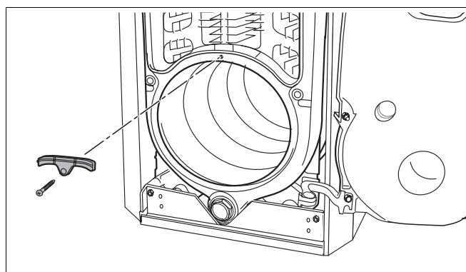
Рис. 71 Удаление стопорной пластины дымовых газов
