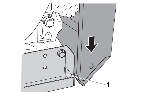
Рис. 45 Установка боковой стенки спереди вниз.
