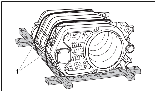
Рис. 31 Котловой блок на палете (вид при поставке)
