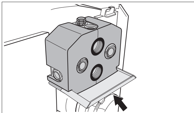
Рис. 52 Установка защитного экрана
