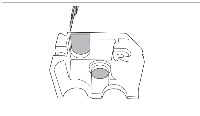
Рис. 50 Вырезание изоляции
