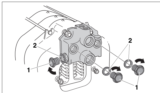
Рис. 25 Установка заглушек в неиспользуемые отверстия
