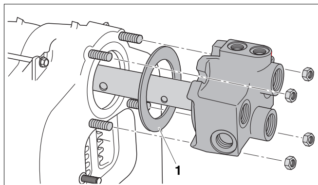
Рис. 23 Установка подпиточной трубы и соединительного элемента
