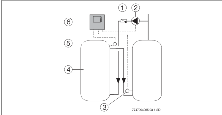
Рис. 4 Функция чередования приоритетности загрузки между двумя водонагревателями
