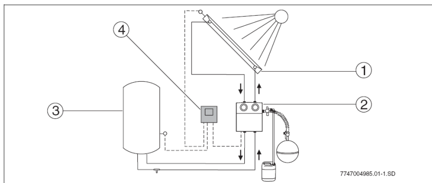
Рис. 2 Схема гелиотермической установки
